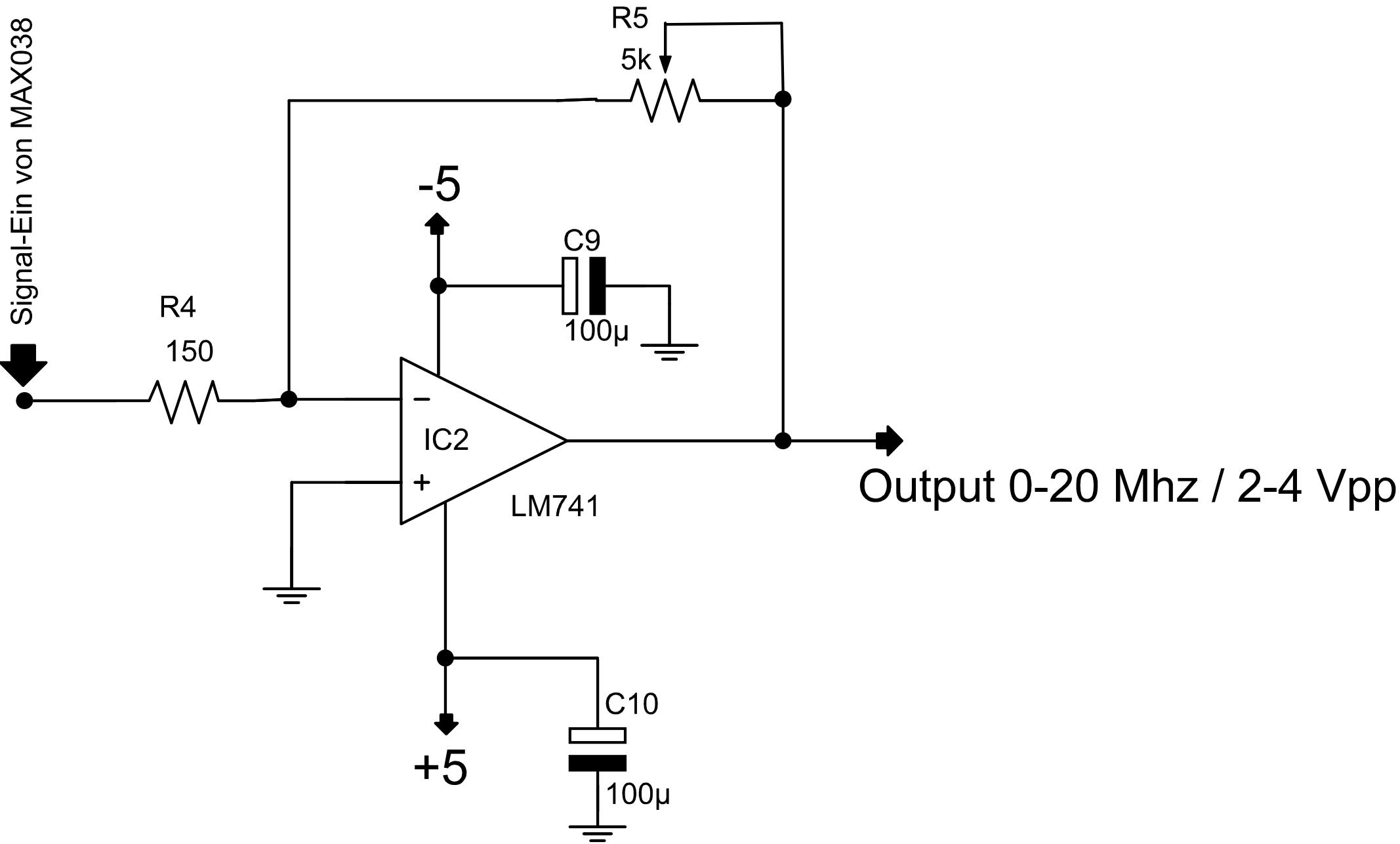
Signal-Ausgangsverstärker für Wobbler MAX038
