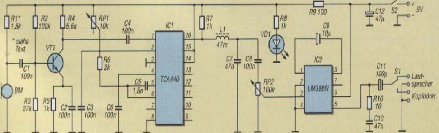
Bild 5: Stromlaufplan des Detektors
